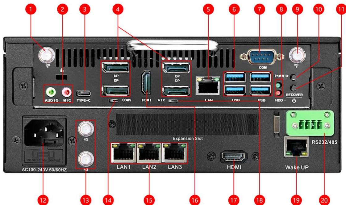
后面板
